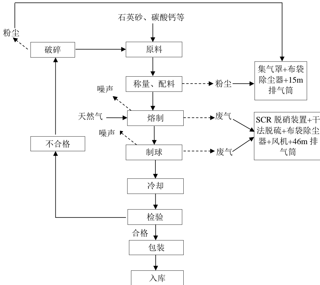
图 2-1 普通无碱玻璃球生产工艺流程及产污环节图
