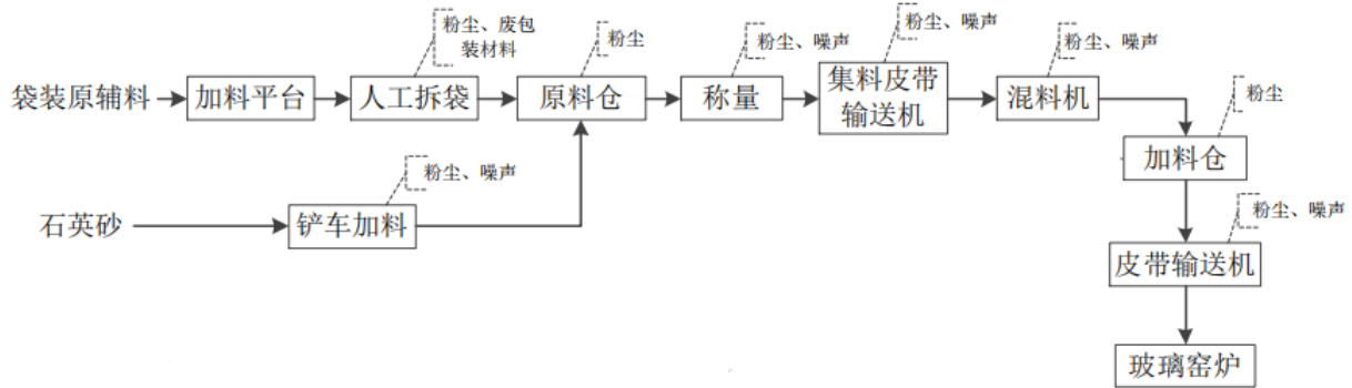
图 2-2 配料混料系统工艺流程及产污环节示意图
